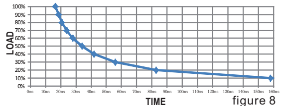
DDR-480D-24
