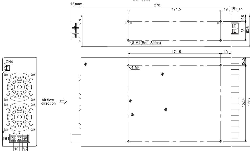
TB1(PFC-450/650/1K0)
