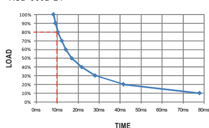
RSD-300B-24
